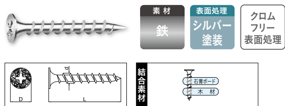
小箱タイプ 頭部梨地
